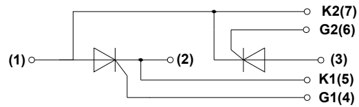
AKMD070
